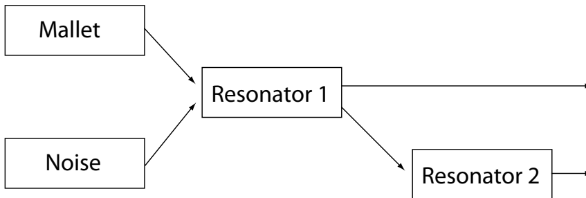
[1 > 2] (直列) 設定の場合の共鳴装置
